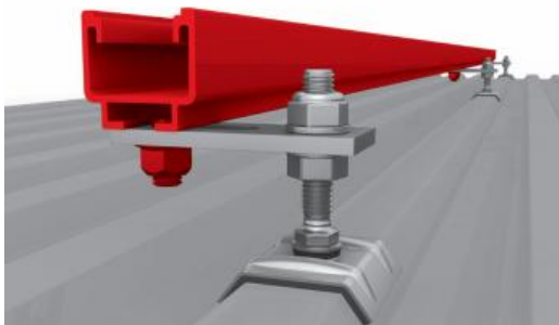
Illustrations de l'assemblage {vis de fixation panneaux solaires + adaptateur + rail 1 ère couche} Gauche : 1 ère couche = SolidRail. Droite : 1 ère couche = SingleRail.
