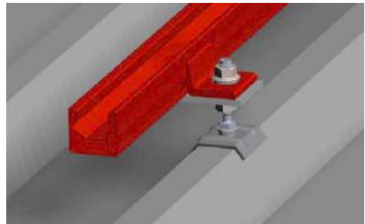
Illustrations de l'assemblage {vis de fixation panneaux solaires + adaptateur + rail 1 ère couche} Gauche : 1 ère couche = SolidRail. Droite : 1 ère couche = SingleRail.
