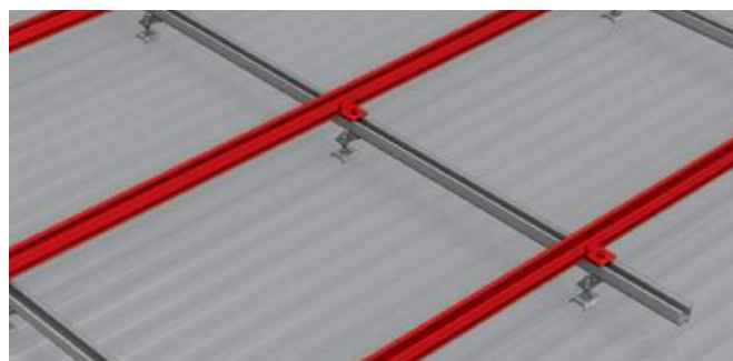
Illustration du procédé K2 SOLIDRAIL SOLARFASTENER PLAQUES NERVURÉES (DROM) (cas de la configuration B)
